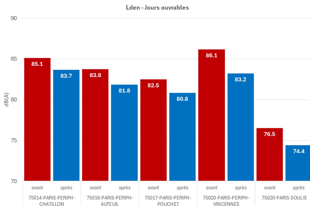
Comparaison des niveaux de bruit selon l'indicateur Lden, exprimés en dB(A), sur les stations du périphérique avant et après l'entrée en vigueur de la baisse de la vitesse limite ; valeurs intégrant la correction liée à la température ; jours ouvrables.
